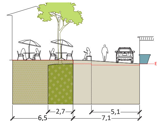
Profil en travers type - Zone de rencontre
