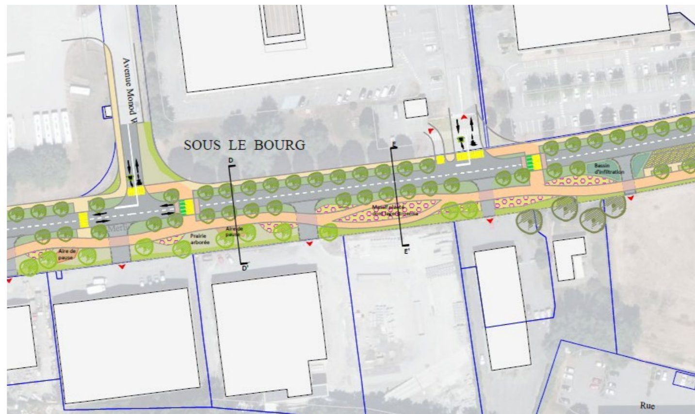
Extrait de plan du scénario retenu - parc linéaire accompagnant l'avenue
