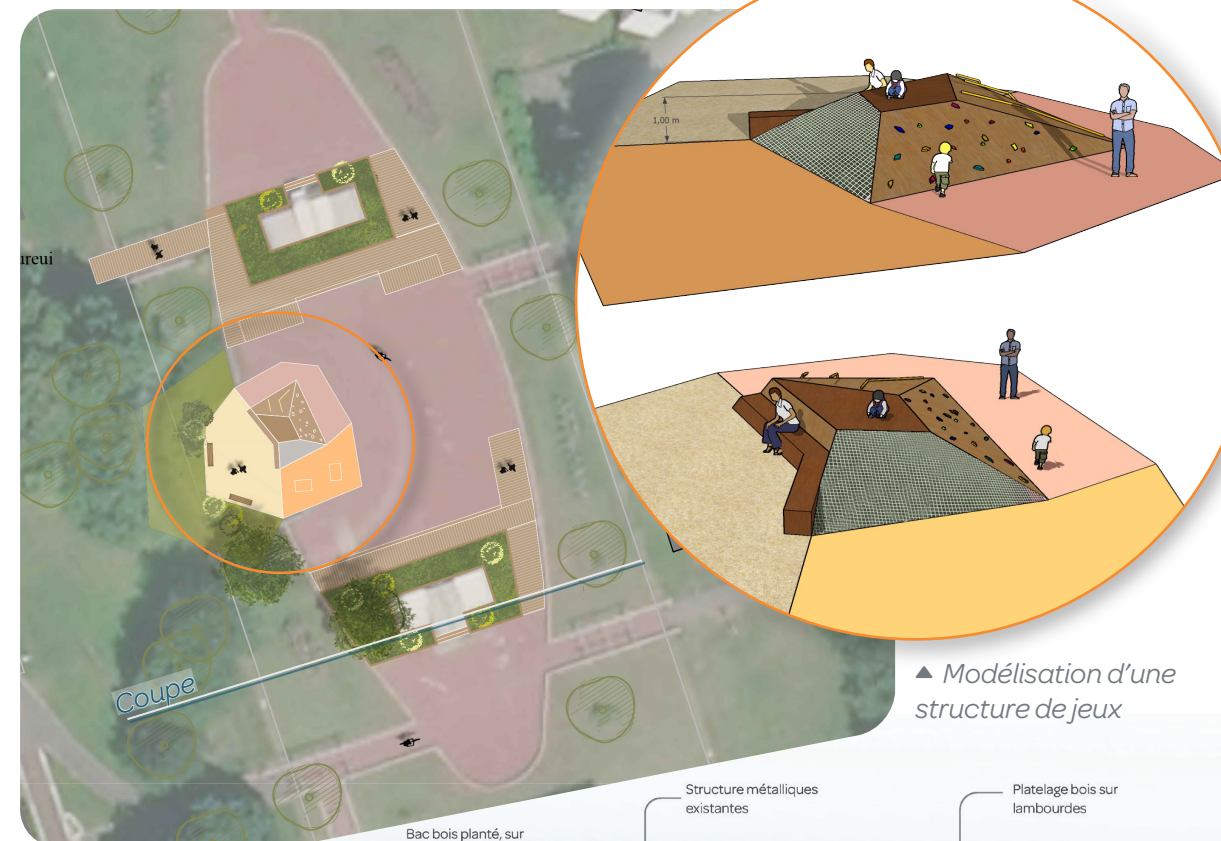
Esquisse d'aménagement pour le quartier de l'Epine ▼
